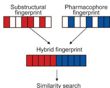
ChemPhysChem DOI: 10.1002/cphc.200900385
