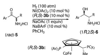
ChemSusChem DOI: 10.1002/cssc.200900128
