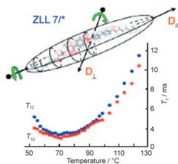
ChemPhysChem DOI: 10.1002/cphc.200900385
